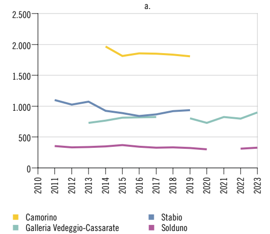
F. 5 VP/giorno feriale, su alcune sezioni della rete stradale, in Ticino, dal 2010
