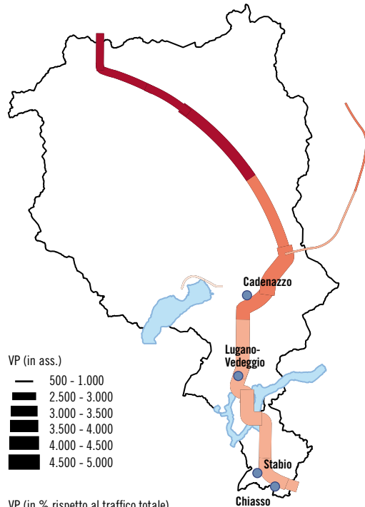
F. 2 VP/giorno feriale (in ass. e in % rispetto al traffico totale), sulla rete autostradale, in Ticino, ultimi dati disponibili*
