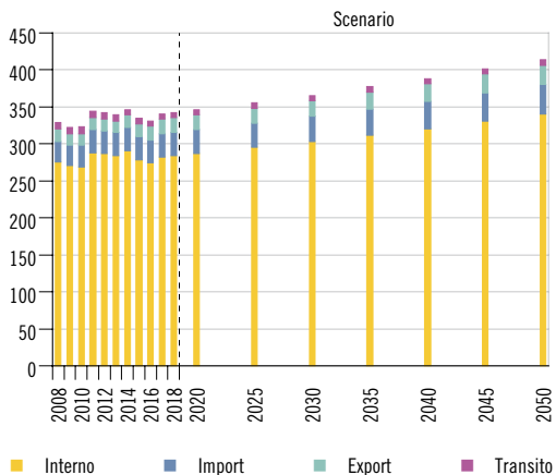
F. 3 Merci trasportate su strada (in mio t), secondo il genere di traffico, in Svizzera: prospettive 2050 (scenario base)
