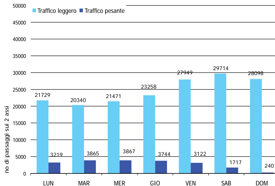
Figura 8: traffico giornaliero medio a Moleno. Numero di passaggi medio nel 2008 sui 2 assi autostradali, suddiviso in traffico leggero e pesante, e ripartito sui singoli giorni della settimana
