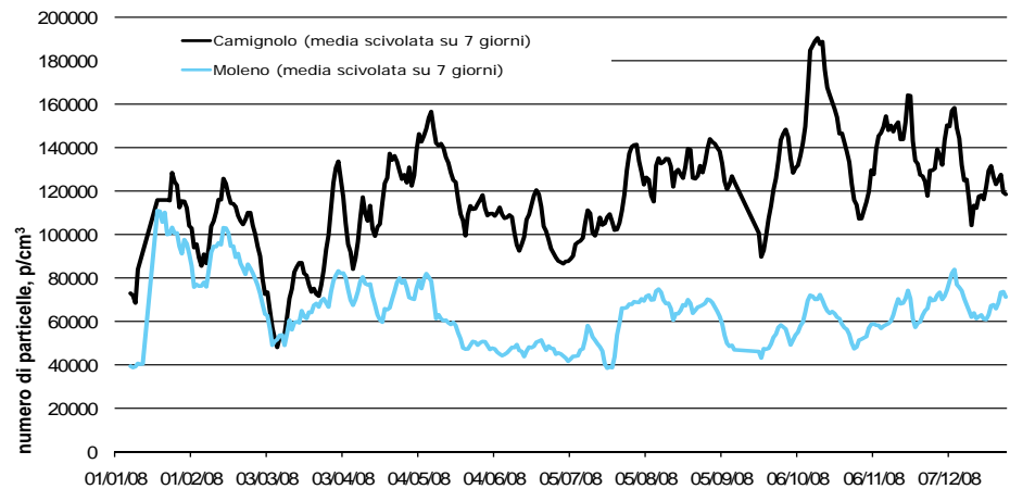
Figura 24: numero di particelle, \text{p}/\text{cm}^3 : andamento annuo, media scivolata su 7 giorni a Moleno e Camignolo, 2008
