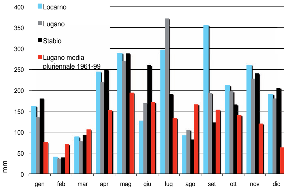
Figura 6.A: somma delle precipitazioni mensili
