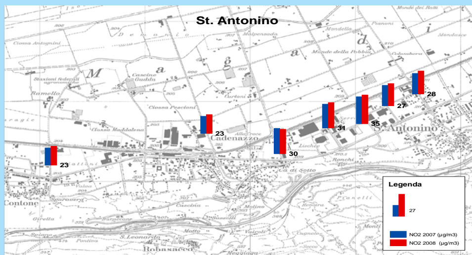
Figura 12: Concentrazioni medie annue di diossido di azoto per il 2007 (blu) e 2008 (rosso) nei dintorni della zona commerciale di S. Antonino. Il valore numerico indica la concentrazione in µg/m 3 nel 2008. (valore limite OIAt per il diossido di azoto: 30 µg/m 3 ).
