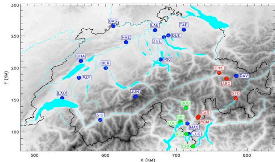
Figura 29: Ubicazione delle stazioni di misura presso utilizzate per valutare i trend dell'ozono
