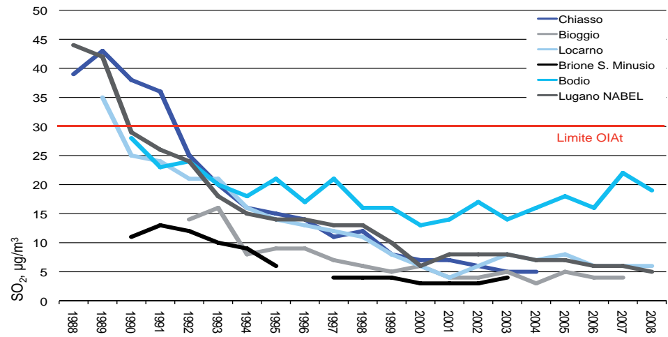
Figura 17: Evoluzione delle medie annue di diossido di zolfo in Ticino, 2008
