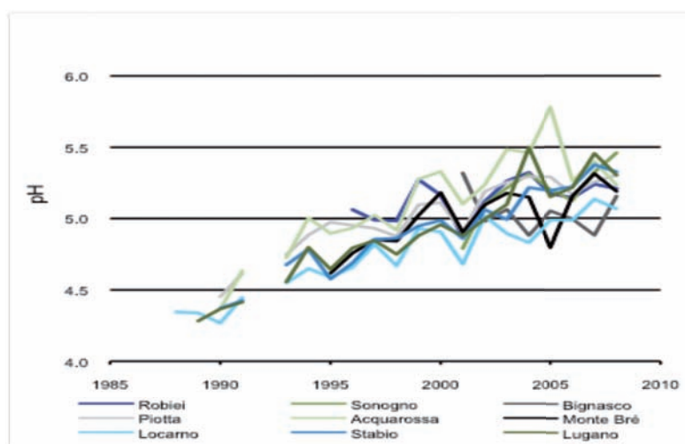
Figura 28: Variazione temporale del pH medio annuo
