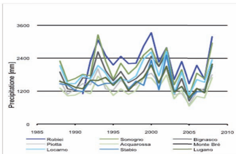
Figura 27: Precipitazione annua; Dati MeteoSvizzera
