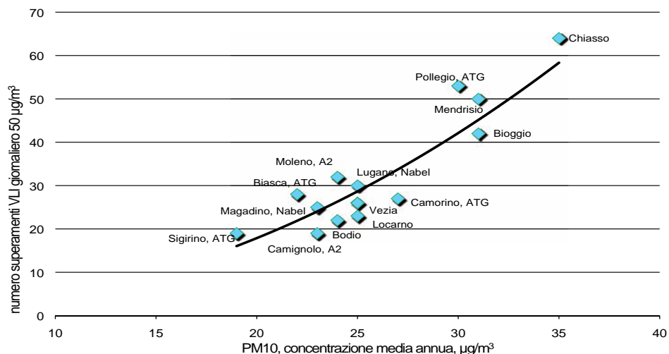
Figura 23: Numero di superamenti del VLI giornaliero in funzione della media annua per le polveri sottili, PM10, in Ticino, 2008
