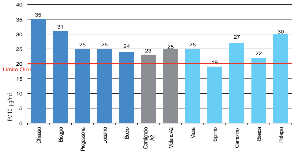
Figura 20: Medie annue delle polveri sottili, PM10, in Ticino, 2008
