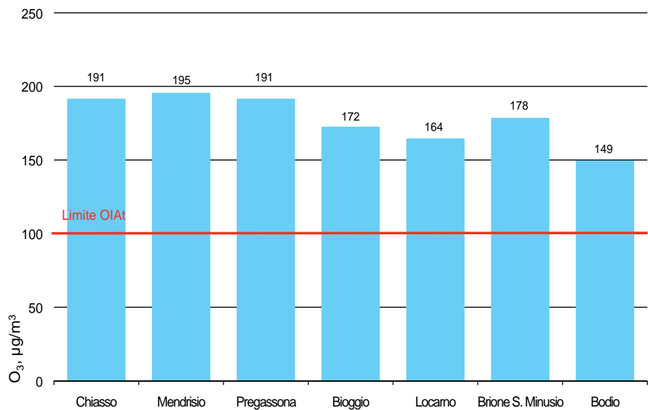
Figura 13: 98° percentile mensile massimo nel 2008
