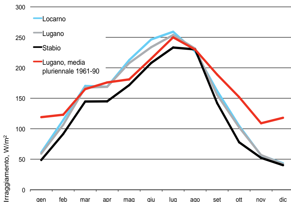
Figura 5.B: irraggiamento, medie mensili
