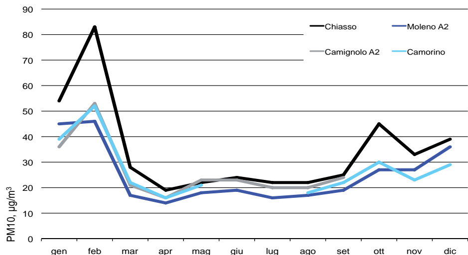
Figura 21: Andamento delle medie mensili delle polveri sottili, PM10, in Ticino, 2008
