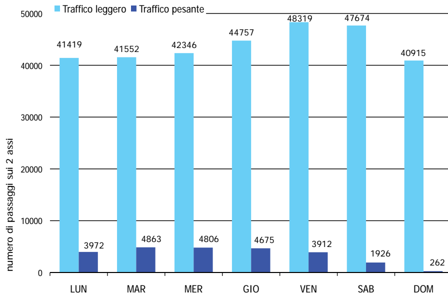
Figura 7: traffico giornaliero medio a Camignolo. Numero di passaggi medio nel 2008 sui 2 assi autostradali, suddiviso in traffico leggero e pesante, e ripartito sui singoli giorni della settimana
