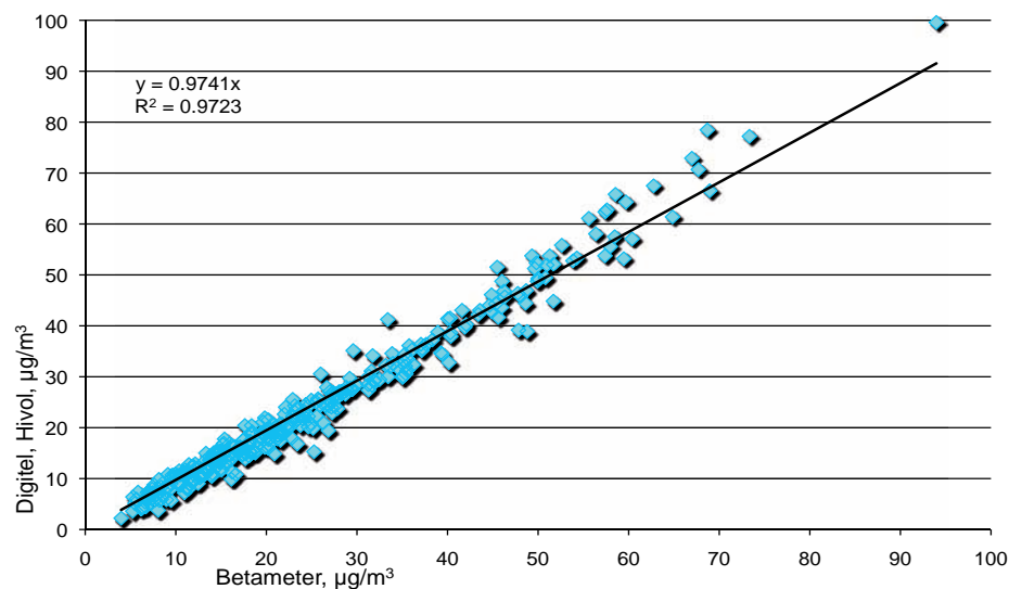
Figura 33: Concentrazioni medie giornaliere di PM10 (periodo gennaio-dicembre 2008) registrate a Camignolo con due metodi di misura diversi (Betameter e Digitel). La linea rappresenta la curva di regressione lineare.
