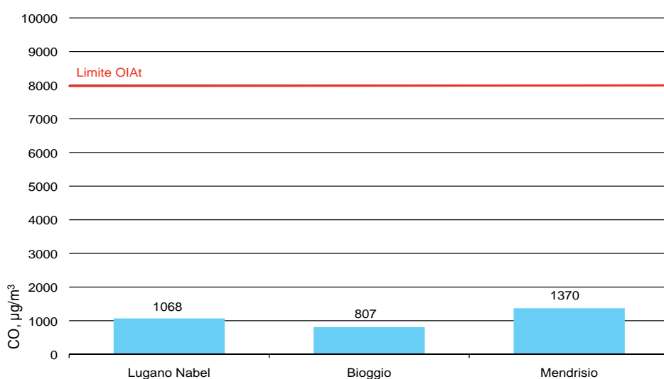
Figura 18: Media giornaliera massima di monossido di carbonio in Ticino, 2008
