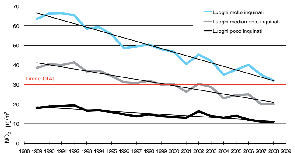
Figura 11: Evoluzione delle medie annue di diossido di azoto in località, poco, mediamente e molto inquinate tramite campionatori passivi, 1989 – 2008
