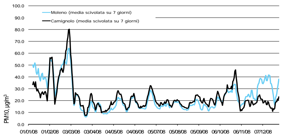
Figura 25: \text{PM}_{10} , \mu\text{g}/\text{m}^3 : andamento annuo, media scivolata su 7 giorni a Moleno e Camignolo, 2008
