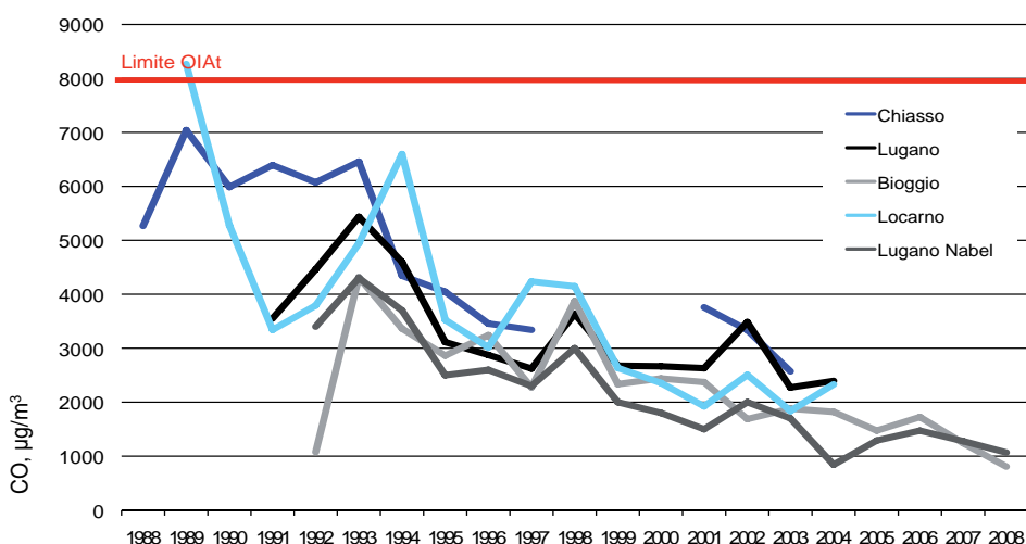
Figura 19: Evoluzione della media giornaliera massima di monossido di carbonio in Ticino, 2008
