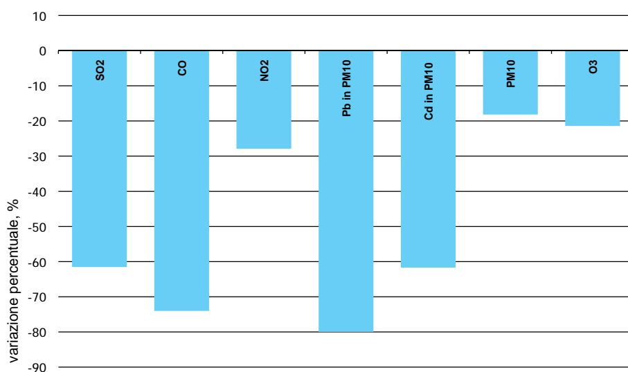
Figura 4: Evoluzione dell'inquinamento atmosferico tra il 1990 e il 2008 per le principali sostanze inquinanti
