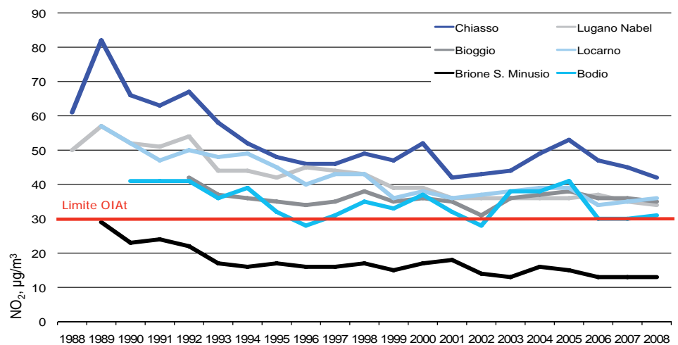
Figura 10: Evoluzione delle medie annue di diossido di azoto in Ticino, 1988 – 2008
