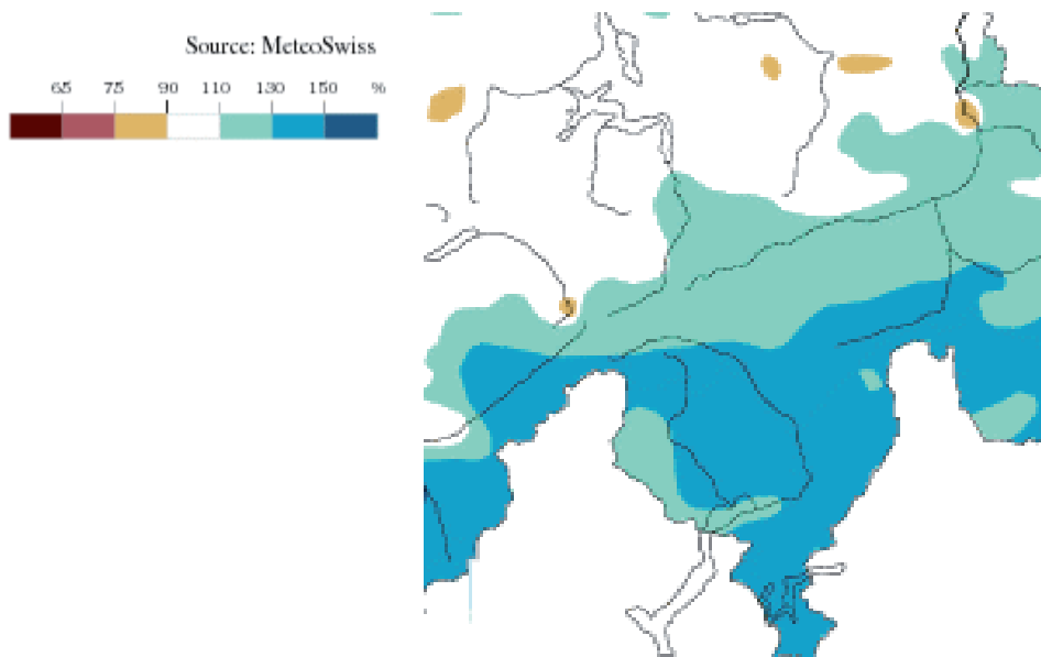
Figura 6.B: deviazione dalla norma delle precipitazioni in Ticino per il 2008
