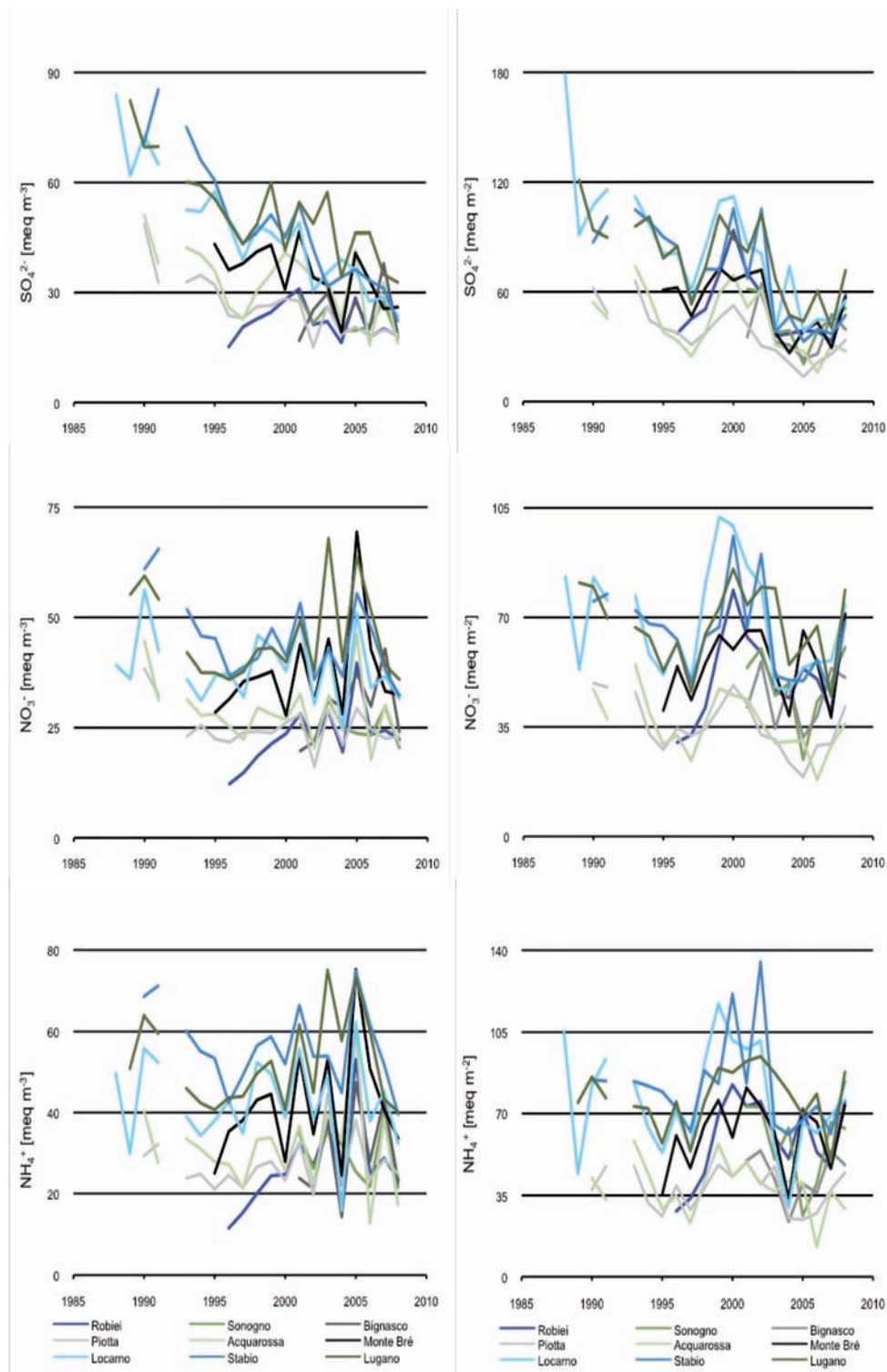
Figura 26: Variazioni temporali delle concentrazioni medie annue (a sinistra), e delle relative deposizioni (a destra) dei principali parametri chimici
