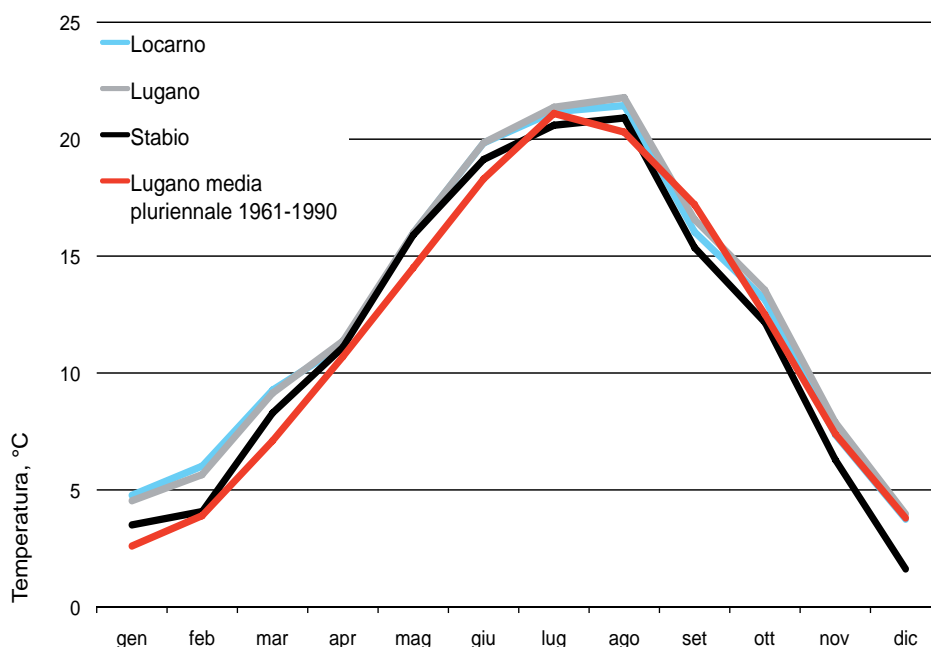
Figura 5.A: temperature, medie mensili
