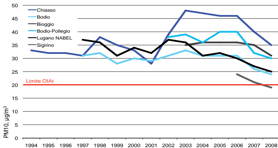
Figura 22: Evoluzione delle medie annue delle polveri sottili, PM10, in Ticino, 1994-2008
