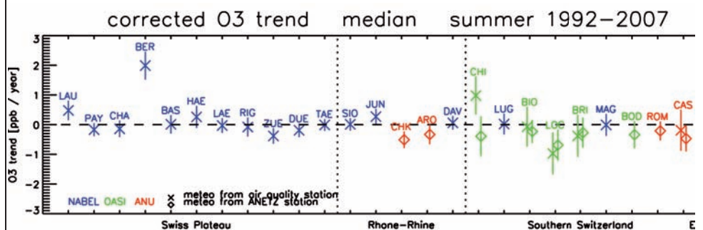
Figura 30: Trend corretti delle mediane di ozono in estate, 1992-2007. Le stazioni delle reti NABEL (blu), OASI/UPA (verde) e ANU (rosso) sono classificate secondo le loro regioni geografiche.
