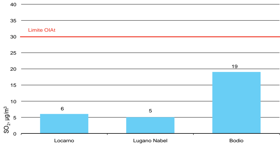
Figura 16: Medie annue di diossido di zolfo in Ticino, 2008
